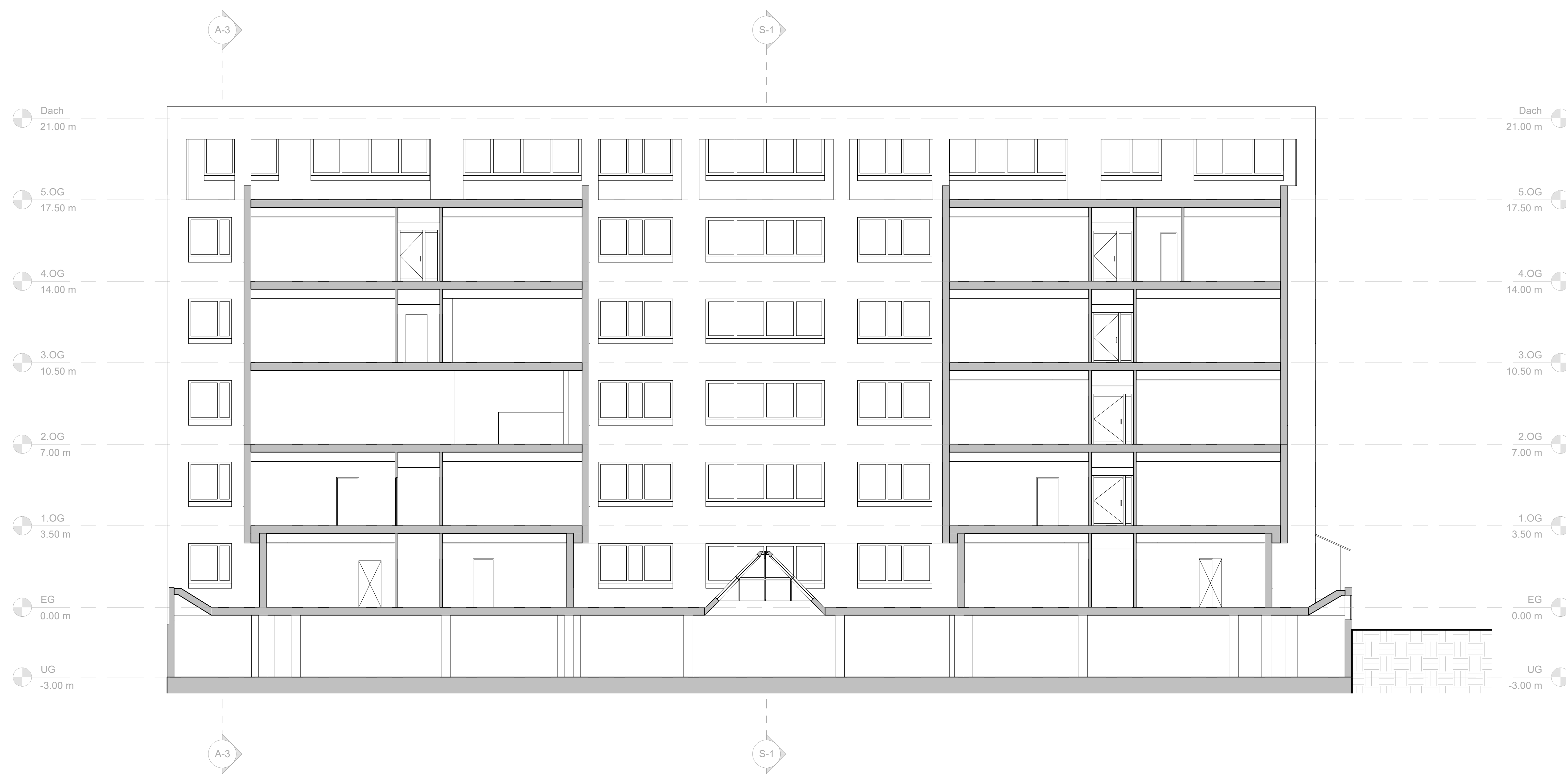
3 Schnitt S-5 1:100
